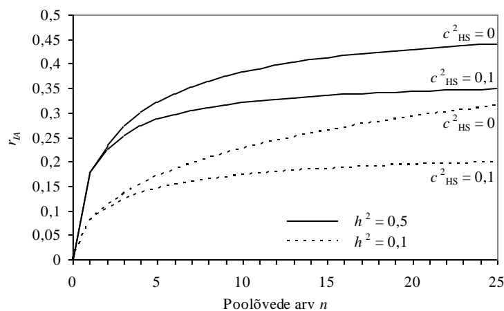
Joonis 3. Poolõvede fenotüübiväärtuste alusel leitud aretusväärtuse hinnangu täpsus sõltuvalt poolõvede arvust, päritavuskoeffitsiendi väärtusest ja poolõvedele ühise mitteaditiivgeneetilise mõju osast.
