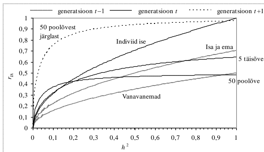
Joonis 4. Aretusväärtuse hinnangu täpsus sõltuvalt päritavuskoefitsiendi väärtusest ja erinevatel ajajärgudel kättesaadavast informatsioonist (püsivad keskkonnaefektid on loetud võrdseks nulliga).
