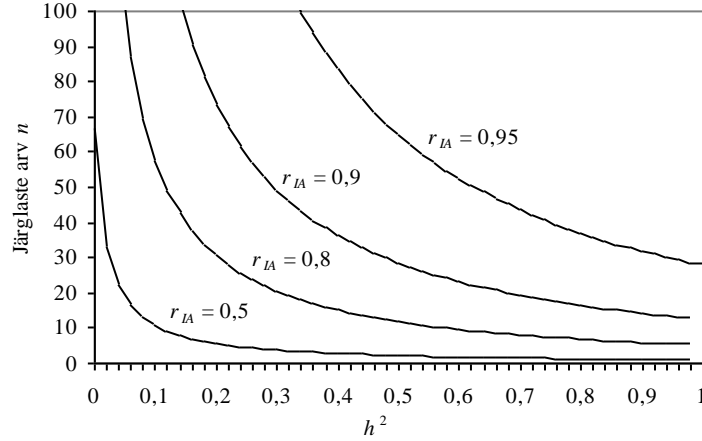
Joonis 2. Isa aretusväärtuse hinnangu täpsus sõltuvalt järglaste arvust ja päritavuskoefitsiendi väärtusest.
