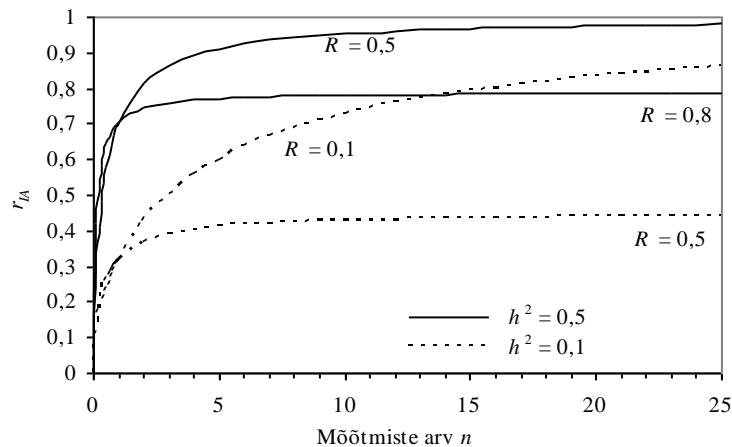
Joonis 1. Indiviidi aretusväärtuse hinnangu täpsus sõltuvalt mõõtmiste arvust ning päritavuskoeffitsiendi ja korduvuse väärtustest.
