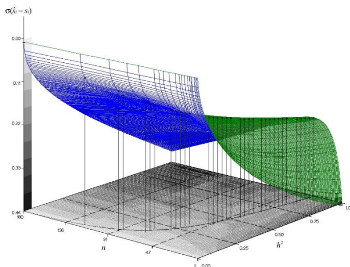
Joonis 1. Isa mõju hinnangu täpsus (mõõdetuna keskmise prognoosiveana \sigma(\hat{s}_i - s_i) ) sõltuvalt järglaste arvust ja päritavuskoeffitsiendi väärtusest vaatluste arvu N = 360 korral. Pidev joon xy -tasandil märgib optimaalset tütarde arvu isa kohta pideval ja vertikaalsed jooned diskreetsel skaalal.
