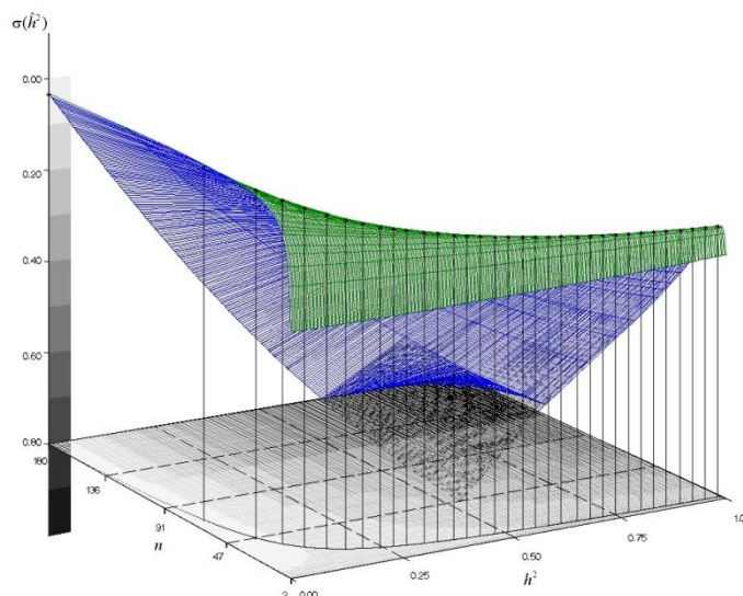
Joonis 2. Päritavuskoeffitsiendi hinnangu täpsus (mõõdetuna hinnangu standardhälbena \sigma(\hat{h}^2) ) sõltuvalt järglaste arvust ja tegelikust päritavuskoeffitsiendi väärtusest vaatluste arvu N = 360 korral. Pidev joon xy -tasandil märgib optimaalset tütarde arvu isa kohta pideval ja vertikaalsed jooned diskreetsel skaalal.
